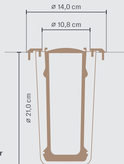
Bohrskizze für Vasenringe
